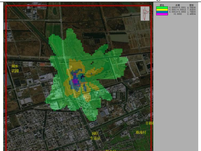
PM 10 日均贡献浓度最大值分布图 ( \text{mg}/\text{m}^3 )
