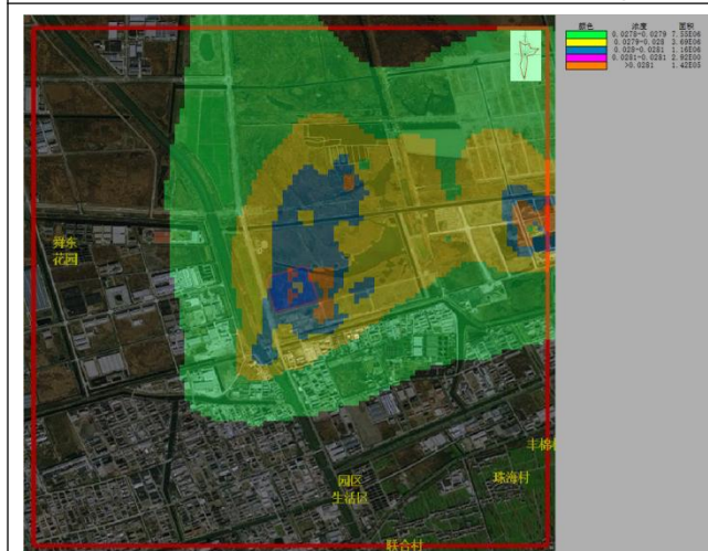
\text{PM}_{2.5} 叠加后年均贡献浓度最大值分布图 ( \text{mg}/\text{m}^3 )
