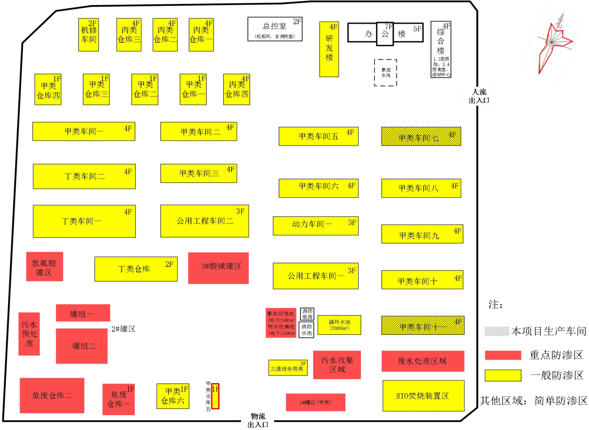
图 7.3-1 企业厂区分区防渗示意图
