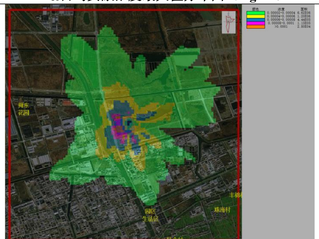
PM 2.5 日均贡献浓度最大值分布图 ( \text{mg}/\text{m}^3 )
