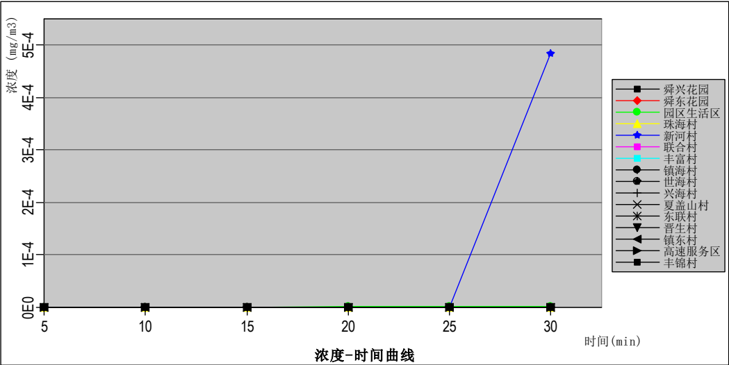
图 6.4.5-12 各关心点处甲苯浓度随时间的变化曲线（最不利气象）
