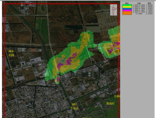
\text{PM}_{10} 叠加后日均贡献浓度最大值分布图 ( \text{mg}/\text{m}^3 )
