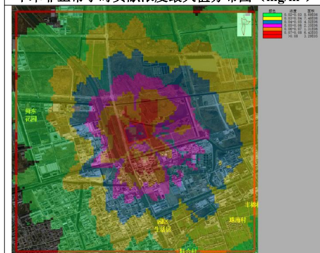
甲醇非正常小时贡献浓度最大值分布图 ( \text{mg}/\text{m}^3 )
