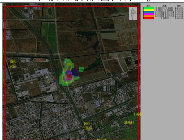
PM 2.5 年均贡献浓度最大值分布图 ( \text{mg}/\text{m}^3 )
