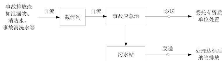
图 6.4.6-3 防止事故废水进入外环境控制、封堵图
