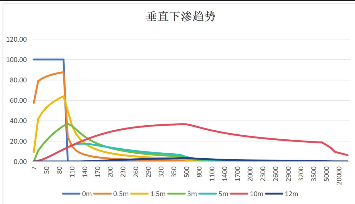
图 6.2.6-1 甲苯垂直下渗土壤污染趋势图
