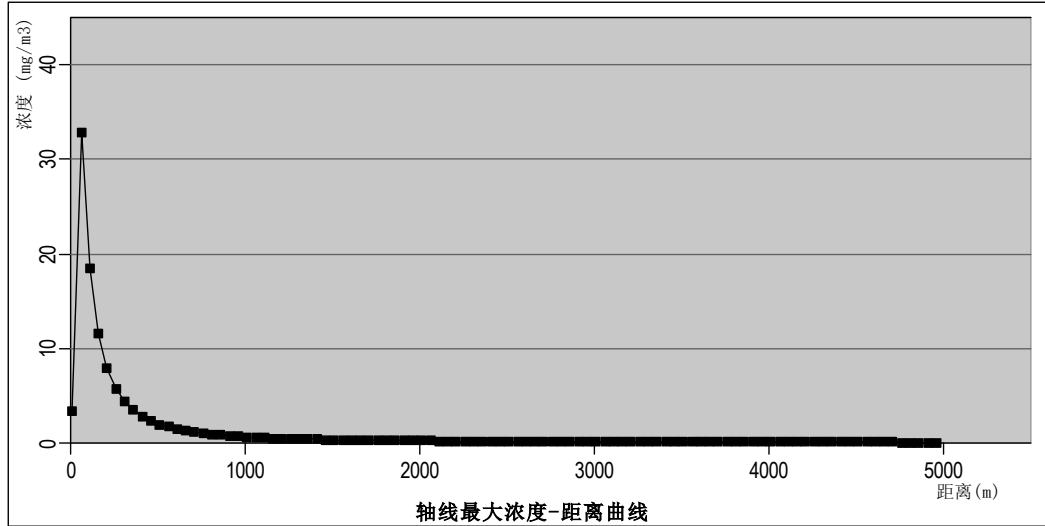
图 6.4.5-4 爆炸 CO 下风向不同距离处最大浓度图（最不利气象条件）
