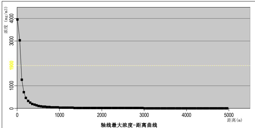
图 6.4.5-16 二氯甲烷泄露下风向不同距离处最大浓度图（最不利气象条件）
