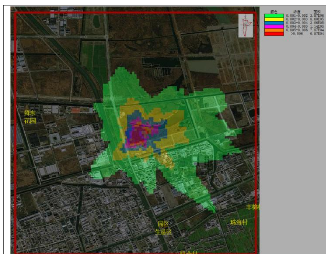
甲醇日均贡献浓度最大值分布图 ( \text{mg}/\text{m}^3 )
