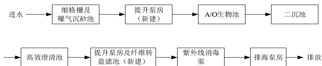
图 2.6-2 绍兴市上虞区水处理发展有限责任公司提标改造工程生活污水处理工艺流程图
