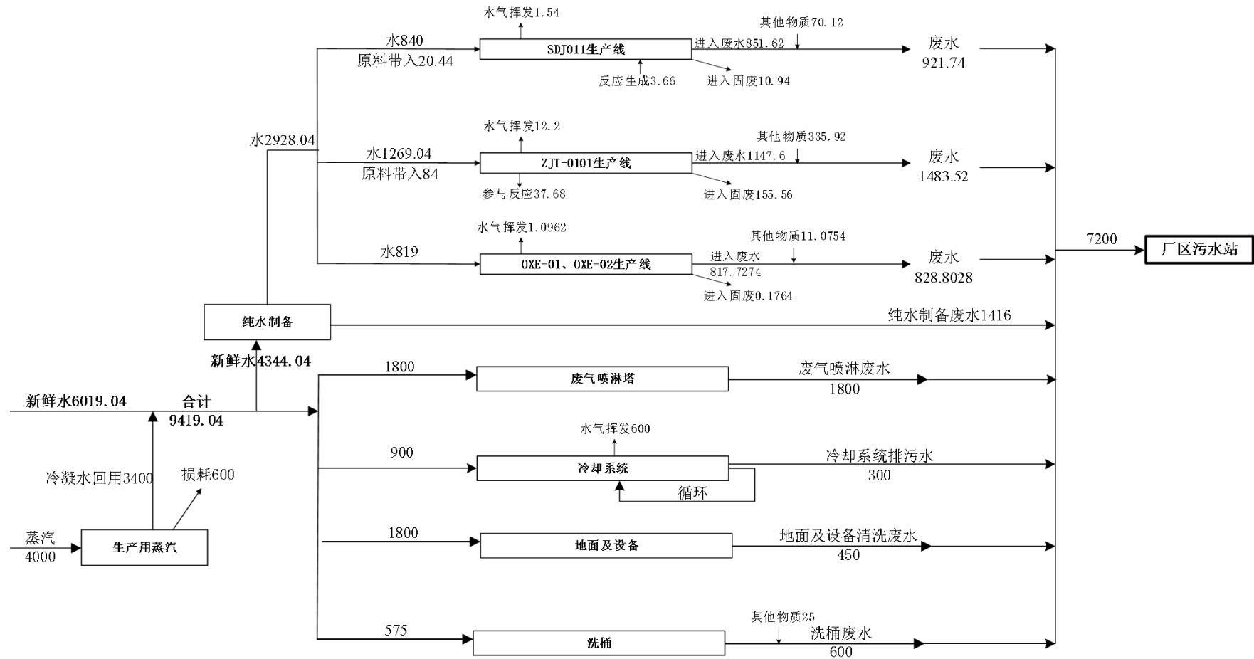
图 4.3-2 项目水平衡图
