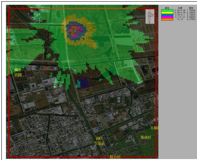
甲苯叠加后小时贡献浓度最大值分布图 (mg/m 3 )
