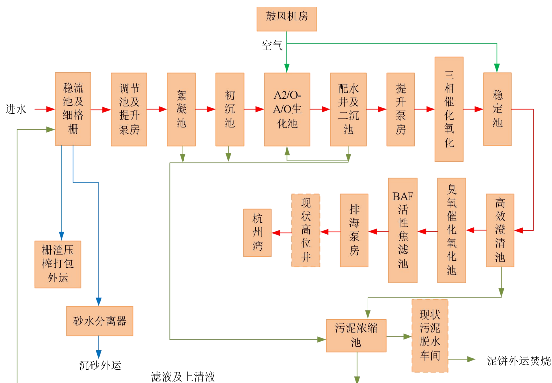
图 2.6-5 绍兴市上虞区水处理发展有限责任公司扩建项目工程污水处理工艺流程图
