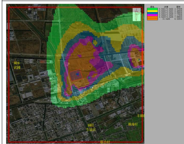
\text{PM}_{10} 叠加后年均贡献浓度最大值分布图 ( \text{mg}/\text{m}^3 )
