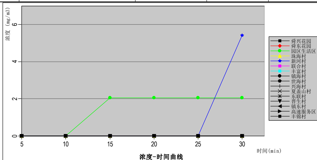
图 6.4.5-18 二氯甲烷泄露浓度随时间的变化曲线（最不利气象）
