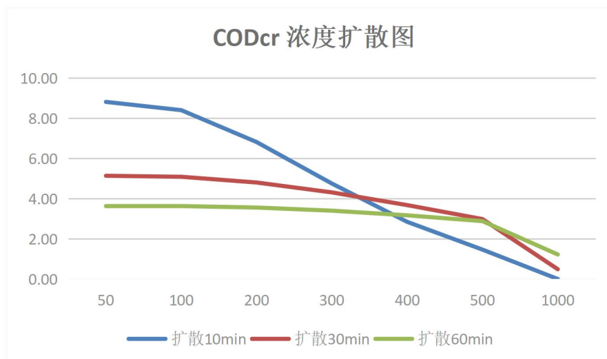
图6.4.5-10 事故废水进入水体中COD Cr 浓度扩散图
