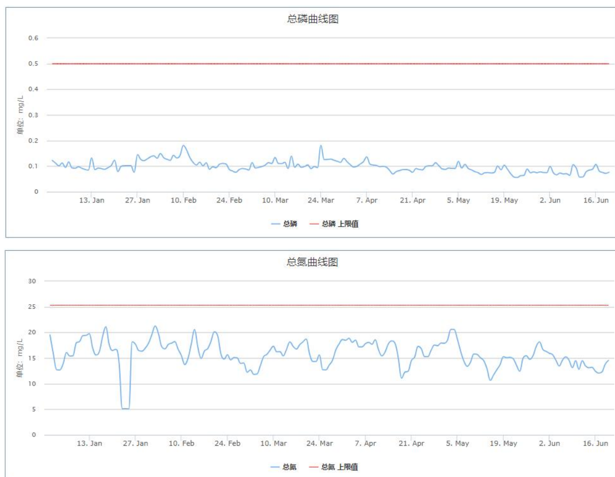
图 2.6-4 绍兴市上虞区水处理发展有限责任公司工业废水处理工程尾水 2025 年 1 月至 6 月监测结果曲线图
