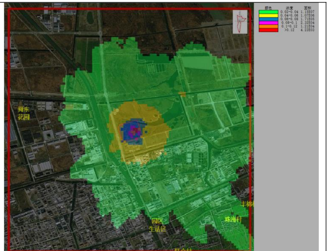
二氯甲烷叠加后小时贡献浓度最大值分布图 (mg/m 3 )
