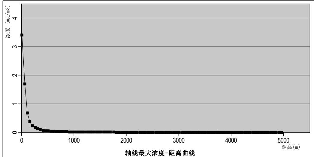
图 6.4.5-10 甲苯泄露下风向不同距离处最大浓度图（最不利气象条件）
