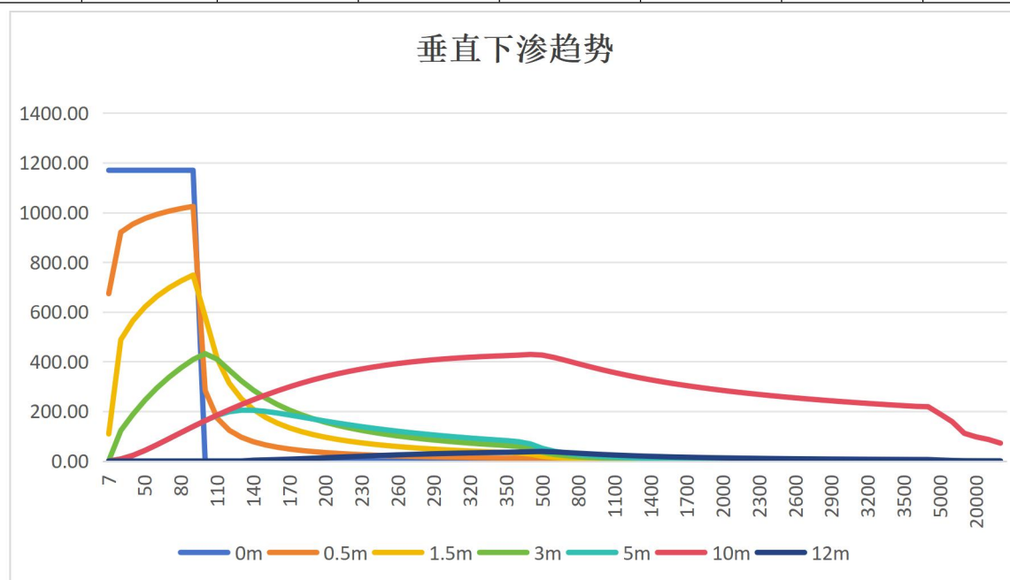
图 6.2.6-2 二氯甲烷垂直下渗土壤污染趋势图
