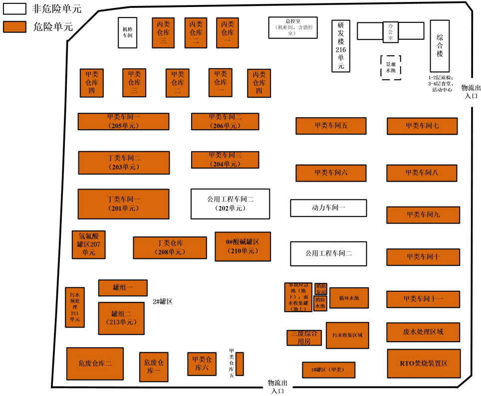
图6.4.4-1 建设项目危险单元分布图
